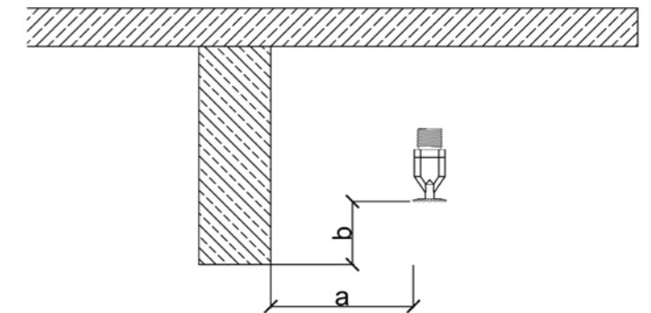
Rys. 7.4. Odległości zraszaczy od belek i podciągów
