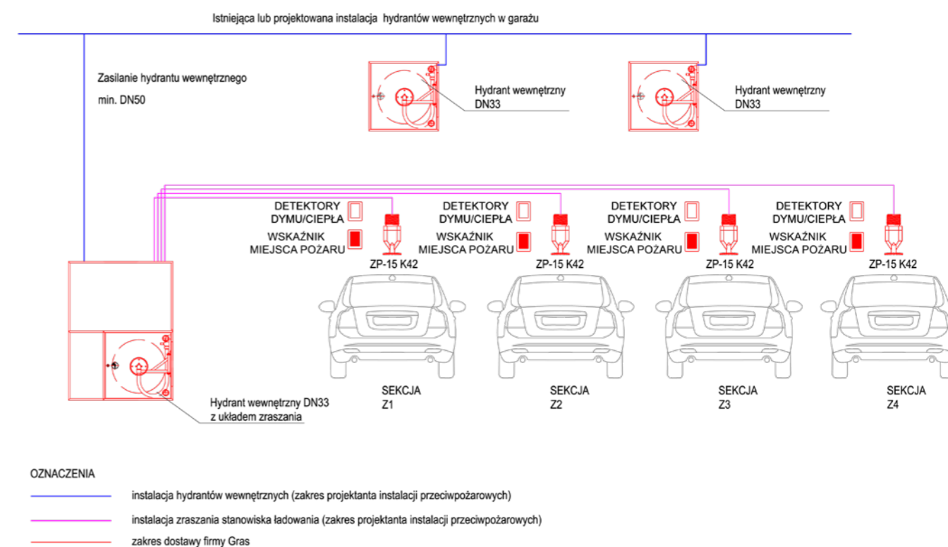
Rys. 7.1. Schemat rozmieszczenia komponentów zestawu hydrantu wewnętrznego z instalacją zraszaczową (komponenty w zakresie dostawy producenta oznaczone na schemacie kolorem czerwonym)
