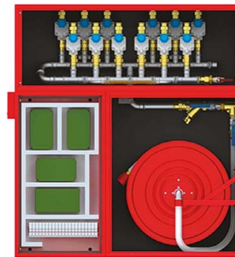
Zestaw hydrantu wewnętrznego z instalacją zraszaczową ZHZ-GN-12 i-Sprink
