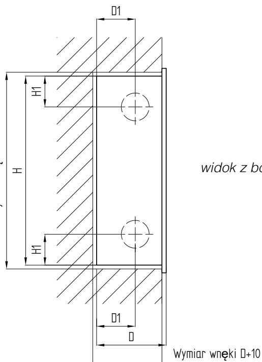
Wymiar wnęki H+20
