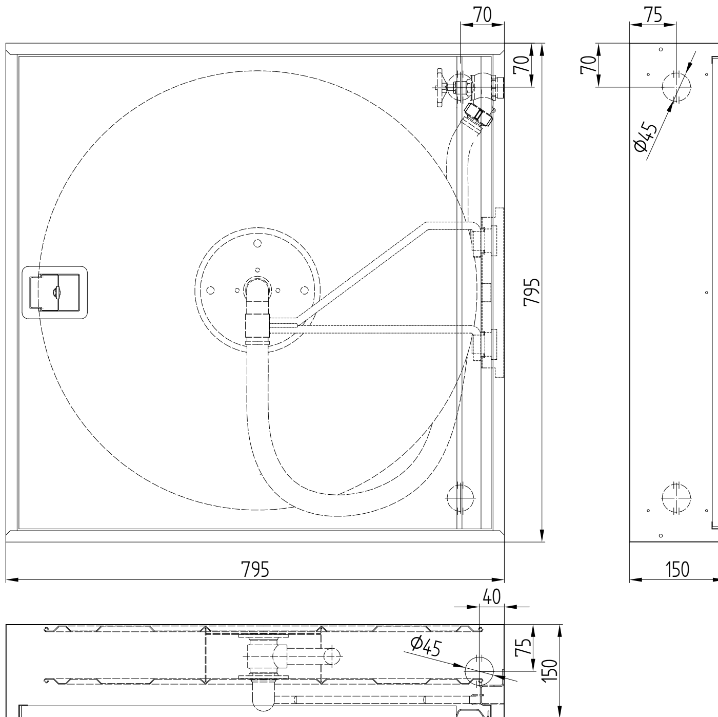
HW-25NW-20/30-SLIM 795x795x150 Wersja nadtynkowa (bez ramek)
