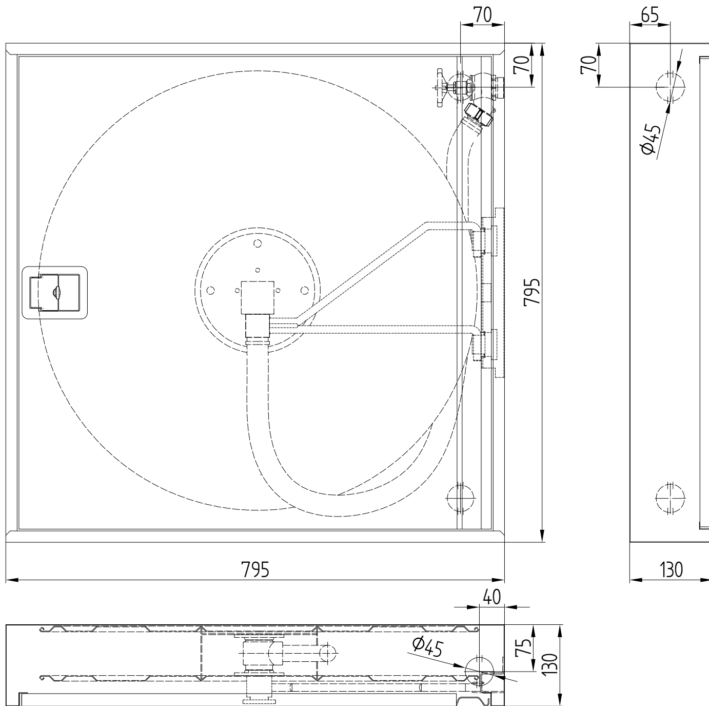
HW-25NW-20/30-SLIM 795x795x130 Wersja nadtynkowa (bez ramek)
